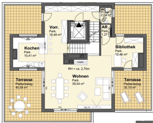
2.DACHGESCHOSS
