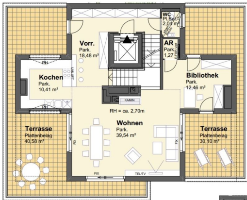
2.DACHGESCHOSS
