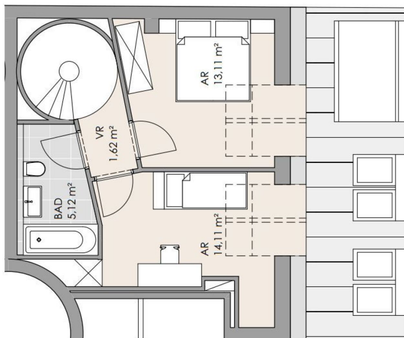
2.DACHGESCHOSS
