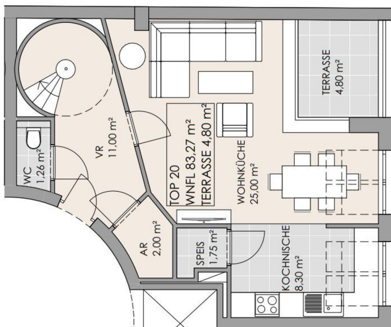
1.DACHGESCHOSS
