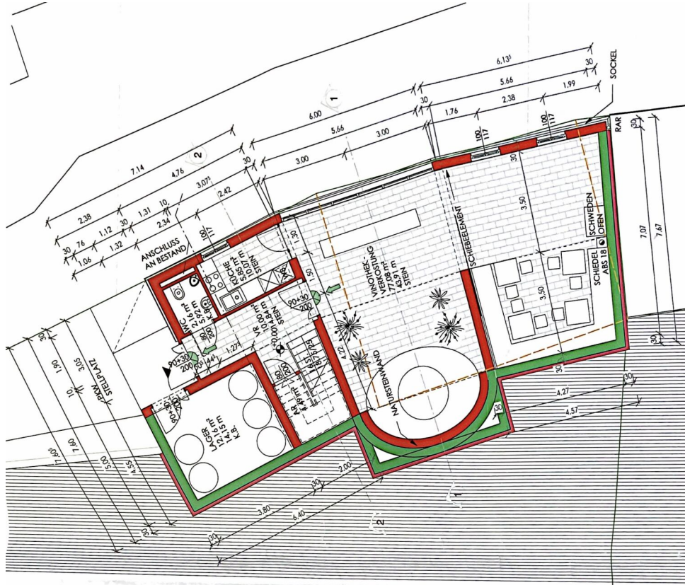
GRUNDRISS EG
