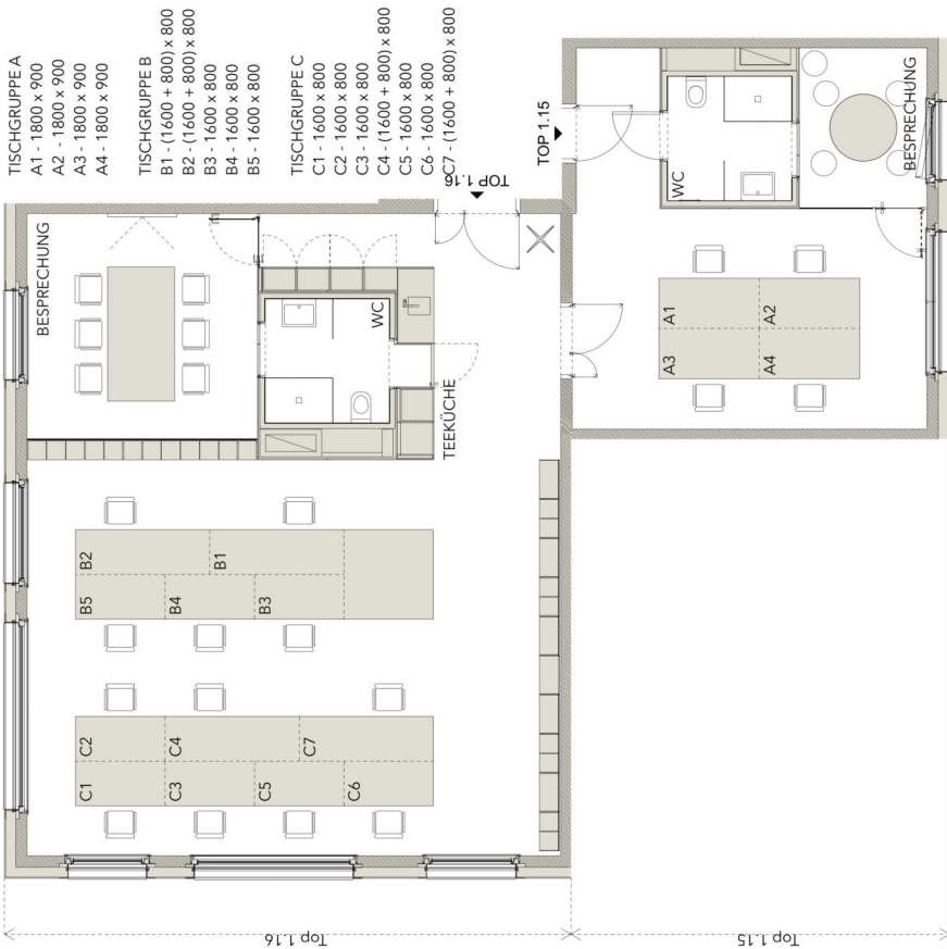
ÜBERSICHTSPLAN ATELIERS 1.15/ 1.16
